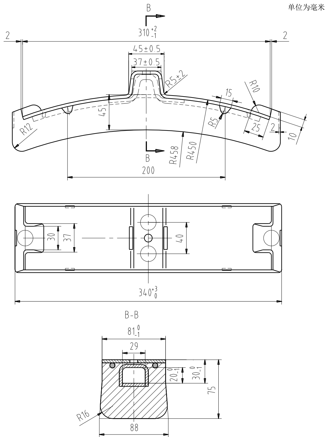
图A.1 闸瓦的型式与主要尺寸
