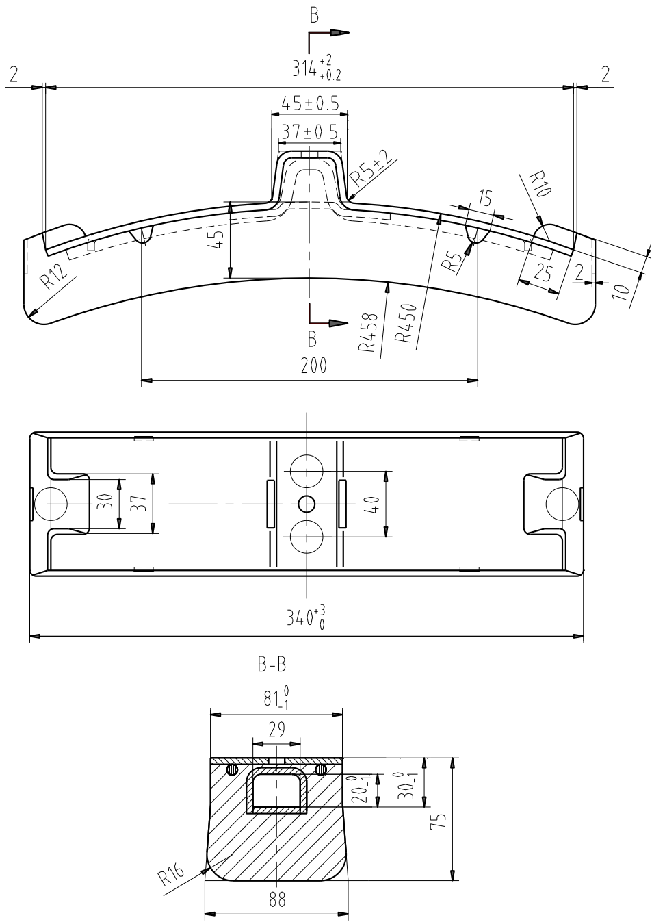
图A. 1 闸瓦的型式与主要尺寸
